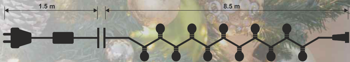
СХЕМА SCHEME схемата се отнася за изделия с размери 8.5м
